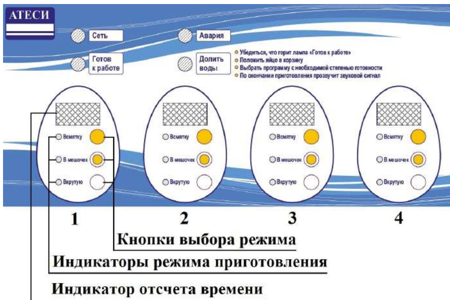
Рис.2 Панель управления.
